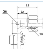
con anello tagliente B4
