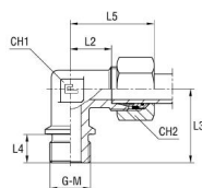
med B4-skärhylsa
