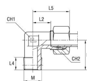
med B3-skärhylsa
