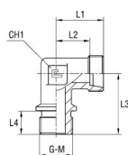
Grundkropp
