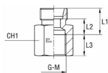
Cuerpo base
