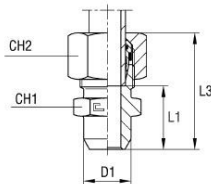
med B4-skärhylsa
