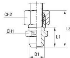
med B3-skärhylsa
