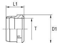
B3-Δακτύλιος κοπής
