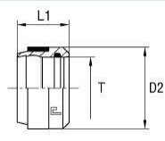
B4-Bague coupante
