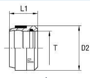
B4-Skärning
