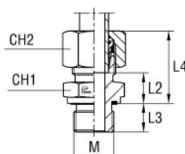
met B4-snijring
