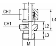
met B4-snijring
