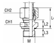
med B3-skärhylsa
