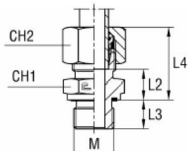
med B4-skärhylsa
