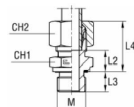
med B3-skärhylsa
