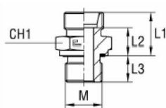
Grundkropp
