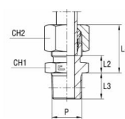
con anello tagliente B3
