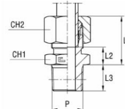
met B3-snijring
