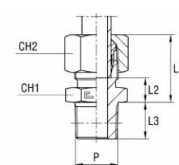
med B3-skärhylsa
