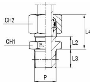
med B4-skärklämring
