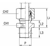
med B4-skärklämring
