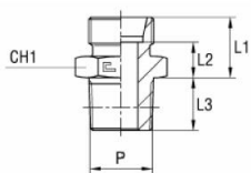
Grundkropp
