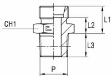
Grundkropp
