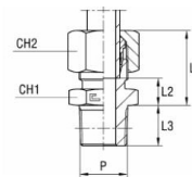
med B3-skärhylsa
