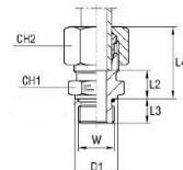
med B3-skæring
