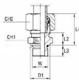
med B4-skæring
