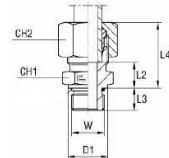
B3-leikkuurengasliitoksella
