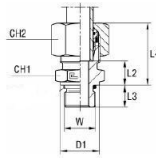
B4-leikkuurenkaalla
