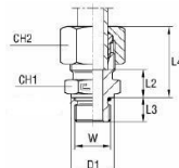
med B3-skjærering
