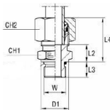
med B4-skjærering
