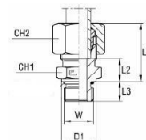
med B3-skärhylsa
