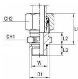
med B4-skärklämring
