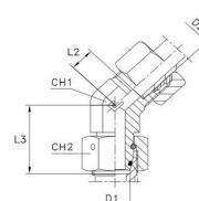
med B3-skärhylsa
