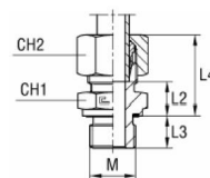
con anello tagliente B3
