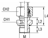
med B4-skärklämring
