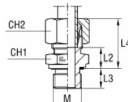
med B3-skärhylsa
