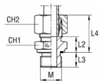
med B3-skärhylsa
