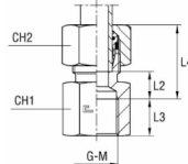
con anillo cortante B4
