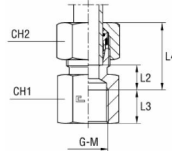
B4-leikkuurenkaalla
