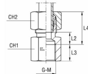
B3-leikkuurengasliitoksella
