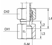
met B3-snijring
