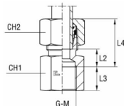
met B4-snijring
