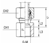
med B4-skärklämring
