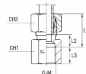
med B3-skärhylsa
