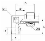
B4-leikkuurenkaalla
