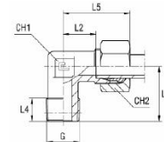
B3-leikkuurengasliitoksella
