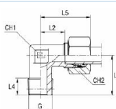
avec bague coupante B4
