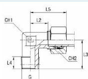
s B4-reznim prstenom
