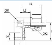
med B3-skärhylsa
