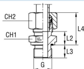
avec bague coupante B4
