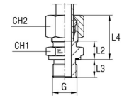
met B3-snijring
