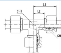
med B3-skärhylsa
