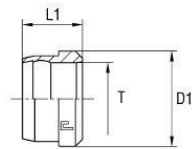
B3-Δακτύλιος κοπής
