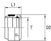
B4-anillo cortante
