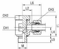
B4-leikkuurenkaalla
