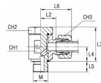
B3-leikkuurengasliitoksella
