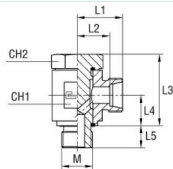
Grundkropp
