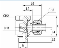
med B4-skärklämring
