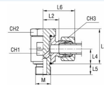
med B3-skärhylsa
