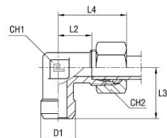
kanssa B3-leikkaurengas
