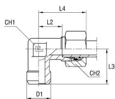
kanssa B4-leikkaurengas
