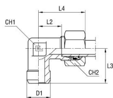
avec bague coupante B4
