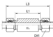
avec bague coupante B4
