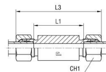
met B3-snijring
