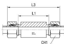
met B4-snijring
