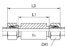
med B4-skärhylsa
