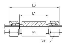
med B3-skärhylsa
