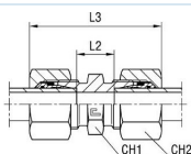
med B4-skärhylsa
