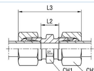
med B3-skärhylsa
