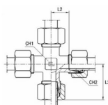
con anillo cortante B4
