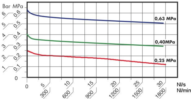
Ingangsdruk = 10bar
