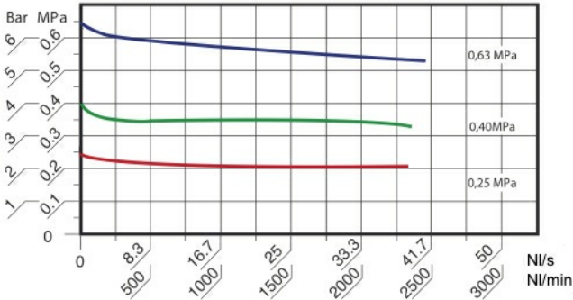
Ingangsdruk = 10bar
