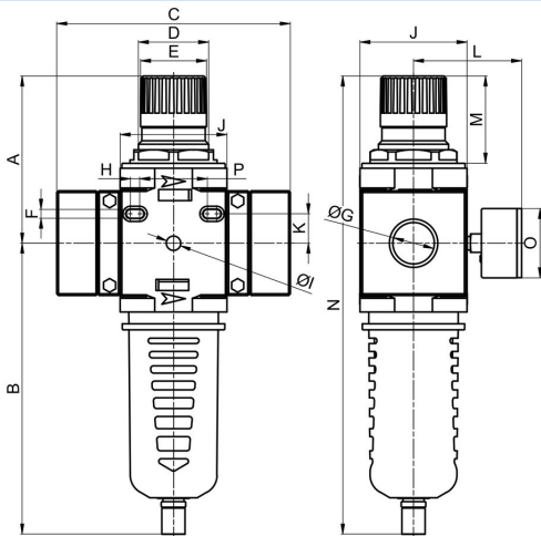
Vægt 0,88kg
