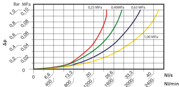
El diagrama muestra diferentes presiones de entrada hasta una caída de presión máx. 1 bar
