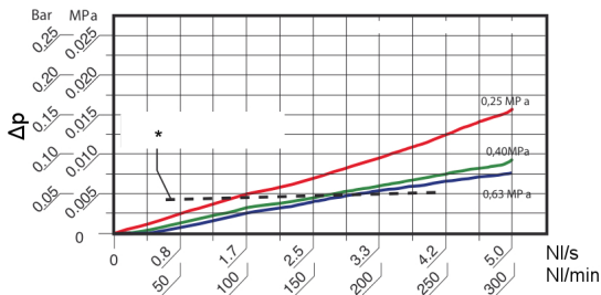
*Debit maxim recomandat Diagrama arată diferite presiuni de intrare
