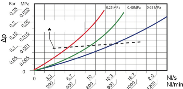
*Anbefalet maksimal gennemstrømning Diagrammet viser forskellige indgangstryk
