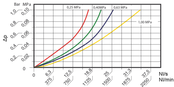
Dijagram prikazuje različite ulazne tlakove do pada tlaka maks. 1bar
